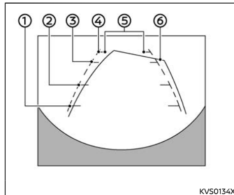
リヤビュー
